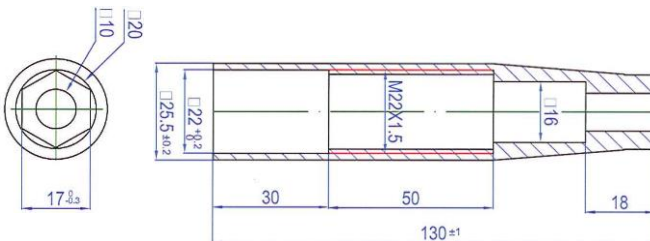
A130L ホイールセンタリングガイドL
