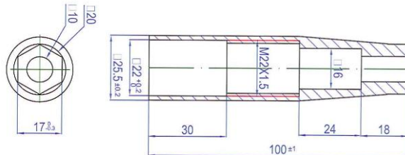
A100S ホイールセンタリングガイドS
